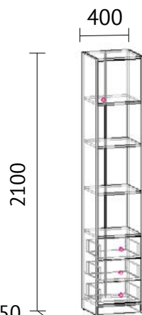
ДМ 1004
