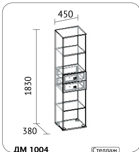
ДМ 1004 (Стеллаж)
