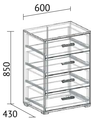
(Комод 600)
