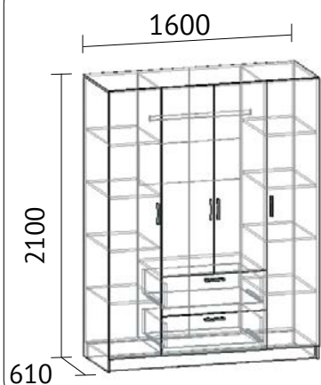
(Шкаф 1.6)
