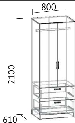
(Шкаф 0.8)
