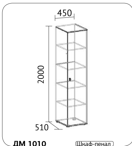
ДМ 1010 (Шкаф-пенал)
